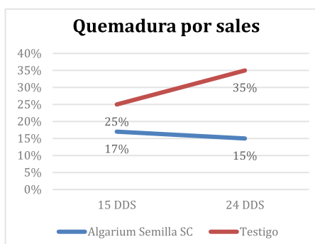
Porcentaje de quemadura por sales con aplicación de Algarium Semilla SC en semillas de maíz blanco
