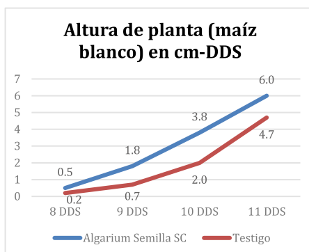
Resultados del efecto de Algarium Semilla SC en el tratamiento de semilla de maíz blanco en bandeja de germinación
